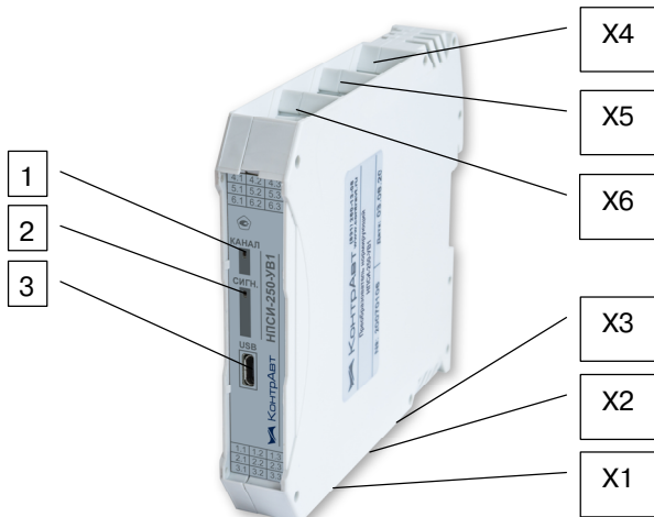
Рисунок 3 – Внешний вид преобразователей HPCH-250/500-UV1.1-xC-24-M(17/ЭМР/xШ/0)
