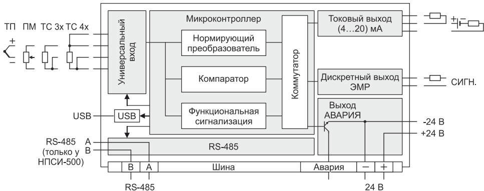
Рисунок 16 – Функциональная структура преобразователей НПСИ-250/500-УВ1.1-1С-24-М(17/ЭМР/1Ш/0)
