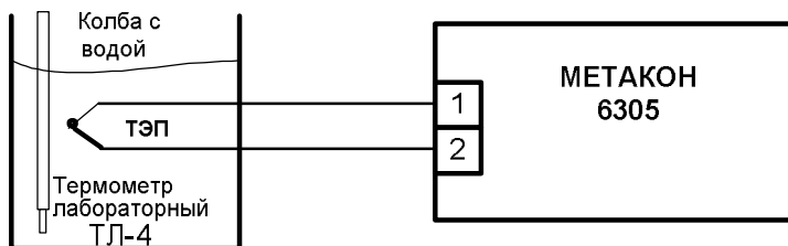
Рисунок А.6.4.2 – Схема проверки погрешности компенсации температуры холодного спая
