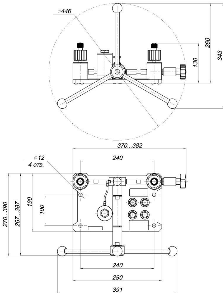
Рисунок 2 – Система гидравлическая ЭЛЕМЕР-СГ-1000-Т (геометрические размеры)
