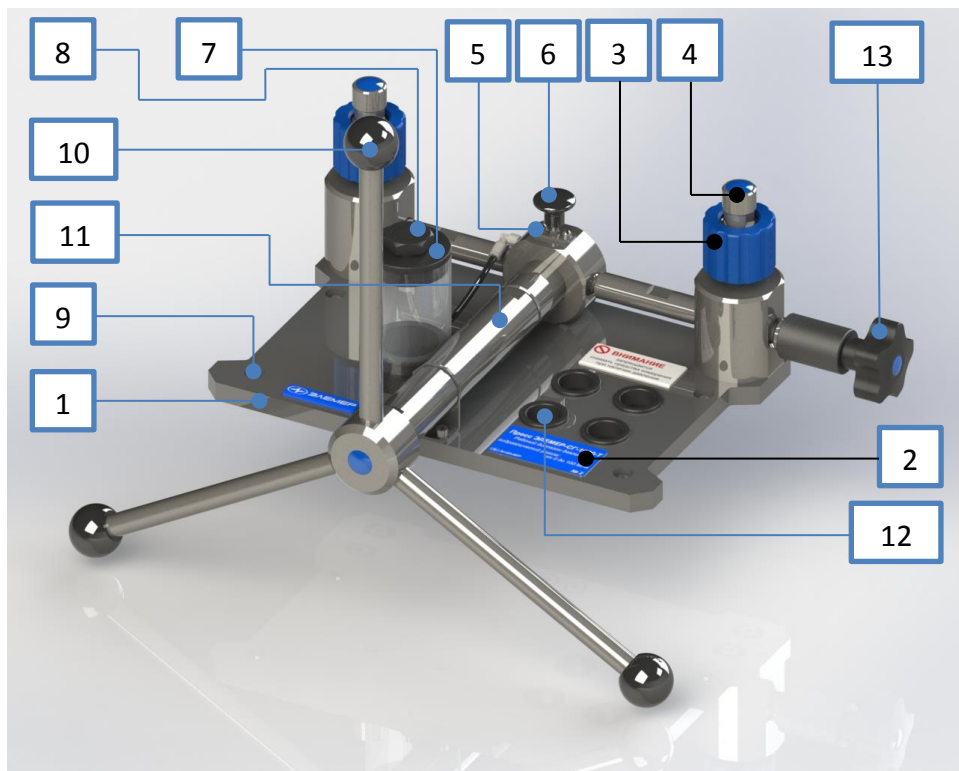
Рисунок 1 – Система гидравлическая ЭЛЕМЕР-SG-1000-T (расположение основных элементов)
