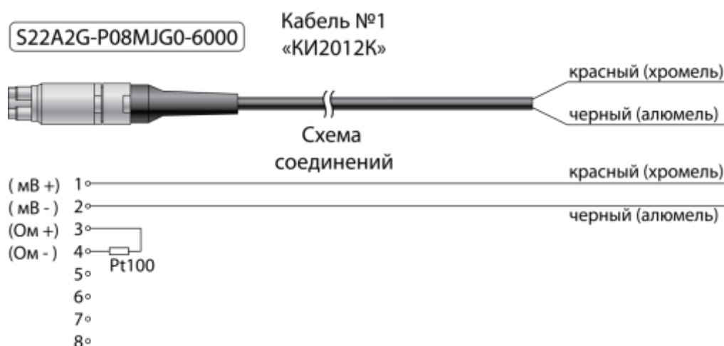
Рисунок А.5 – Соединительный кабель «КИ2012К» для подключения к ИКСУ ТП типа ТХА при работе в режиме измерения температуры, а также для связи с устройствами в режиме воспроизведения сигналов от указанного типа ТП
