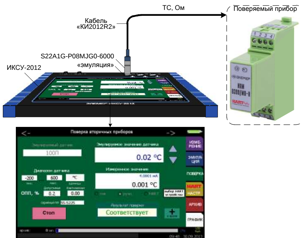
Рисунок 2.83 – Проверка вторичных приборов
