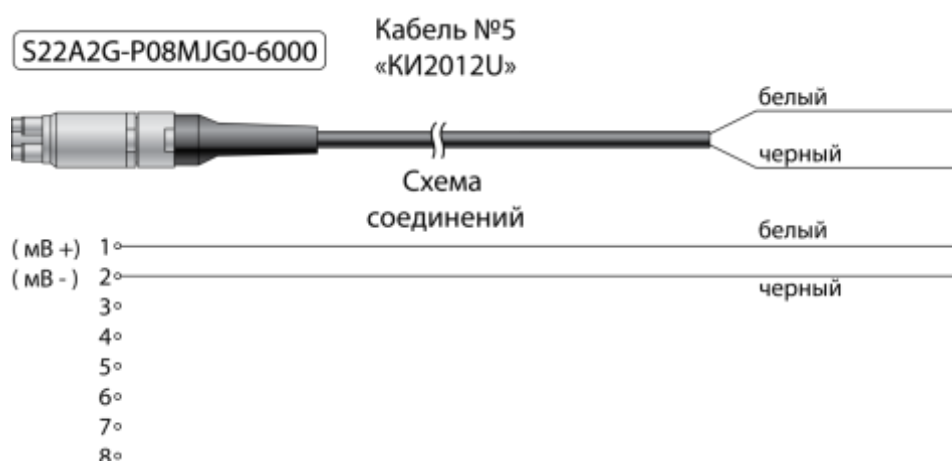
Рисунок А.9 – Соединительный кабель «КИ2012U» для связи ИКСУ с первичными преобразователями или устройствами при работе в режиме измерений напряжения постоянного тока, а также воспроизведения сигналов напряжения постоянного тока
