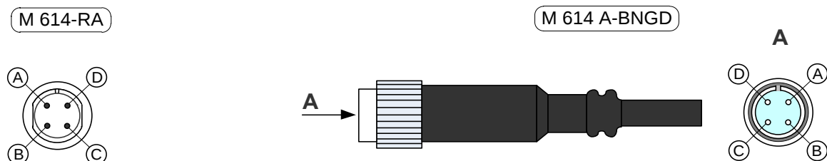
Рисунок А.4 – Разъем для подключения к ПДЭ, ТЦЭ
