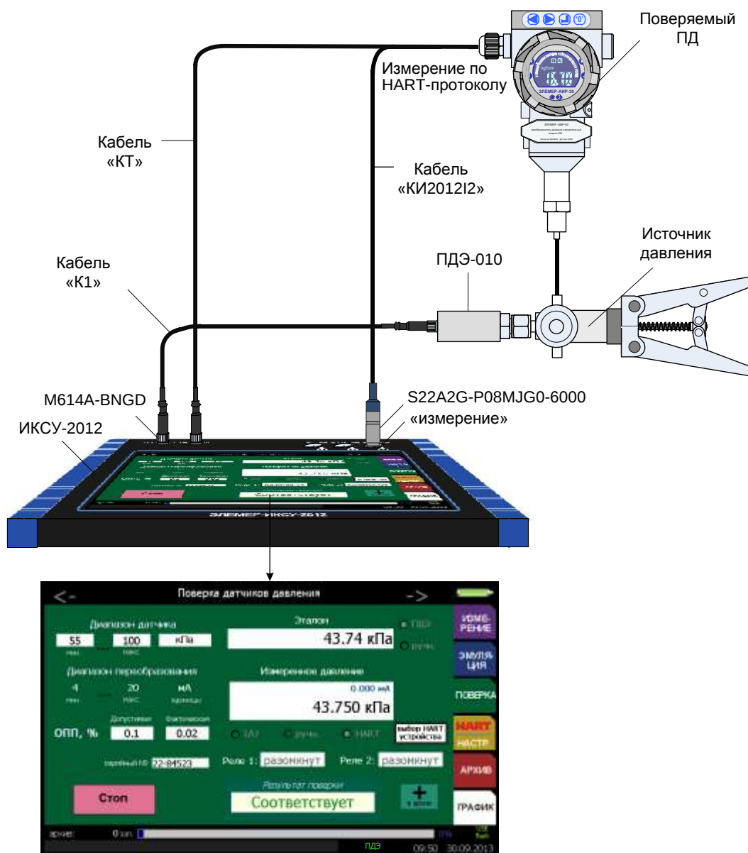
Рисунок 2.87 – Поверка датчиков давления
