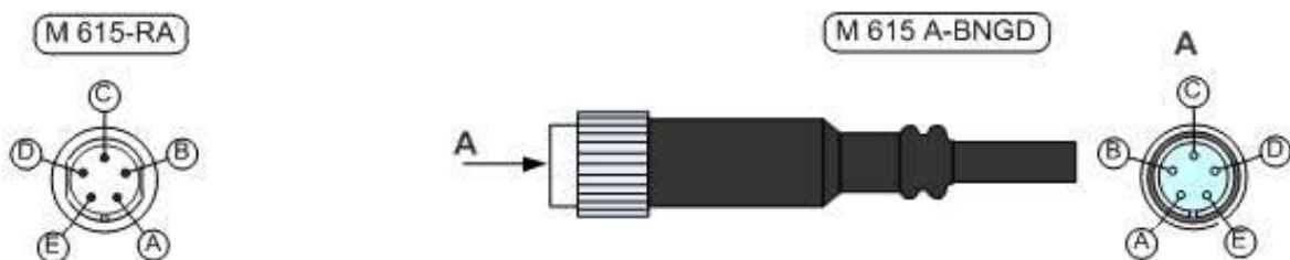
Рисунок А.3 – Разъем для подключения к реле
