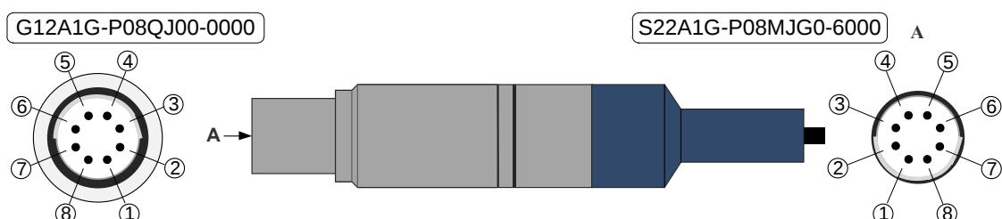
Рисунок А.2 – Разъемы для воспроизведения сигналов от ТС, Ом
