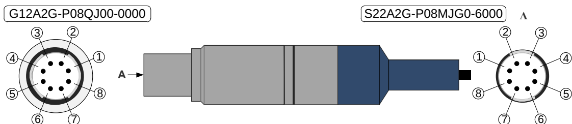
Рисунок А.1 – Разъемы для измерения сигналов от ТП, мА, мВ, В; ТС, Ом и воспроизведения сигналов от ТП, мА, мВ, В
