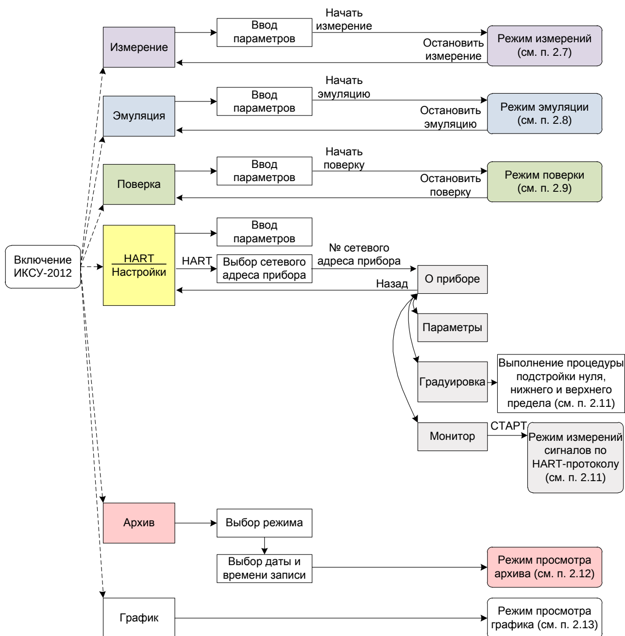
Рисунок 2.5 – Структура меню
