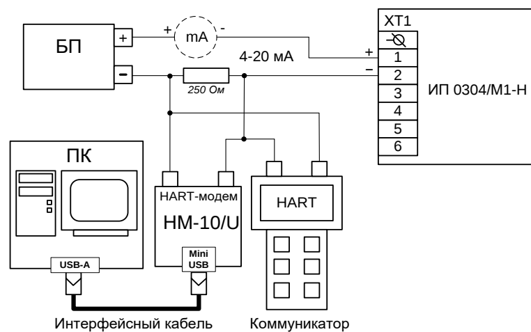
Рисунок А.9 - Схема электрическая подключений ТПУ 0304/М1-Н по HART-протоколу через кабельный или сальниковый ввод
