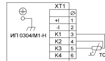
Рисунок А.3 – Подключение сопротивления к ИП 0304/М1-Н, трёхпроводная схема
