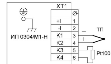
Рисунок А.1 – Подключение термопары к ИП 0304/М1-Н
