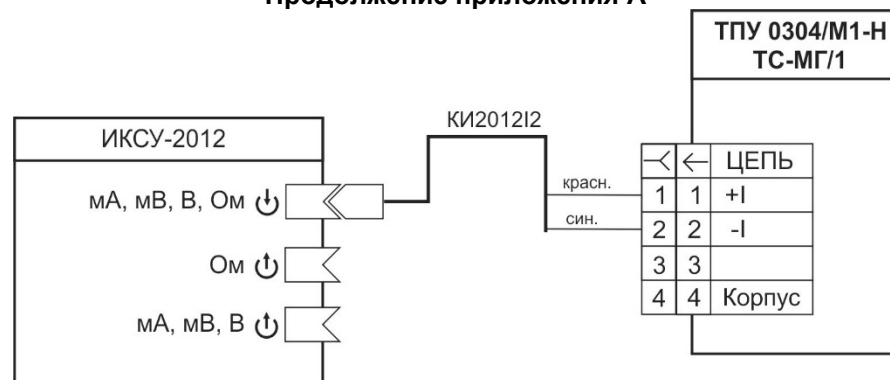
Рисунок А.21 - Схема электрическая подключений ТПУ 0304/M1-H с ПП ТС-МГ/1 с ТС-МГ/1 к ИКСУ
