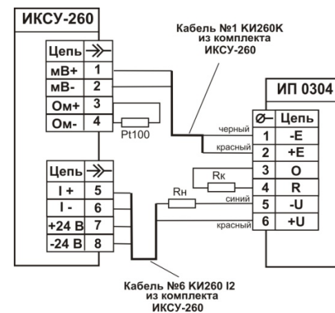
Рисунок А.16 – Схема электрическая подключений ИП 0304/М1-Н и ИКСУ
