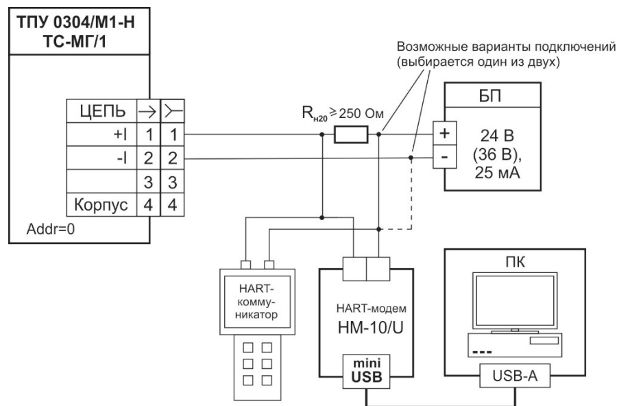
Рисунок А.19 - Схема электрическая подключений ТПУ 0304/M1-H с ТС-МГ/1 по HART-протоколу по схеме «точка-точка» (короткий адрес = 0)
