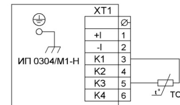
Рисунок А.2 – Подключение термометра сопротивления к ИП 0304/М1-Н, двухпроводная схема
