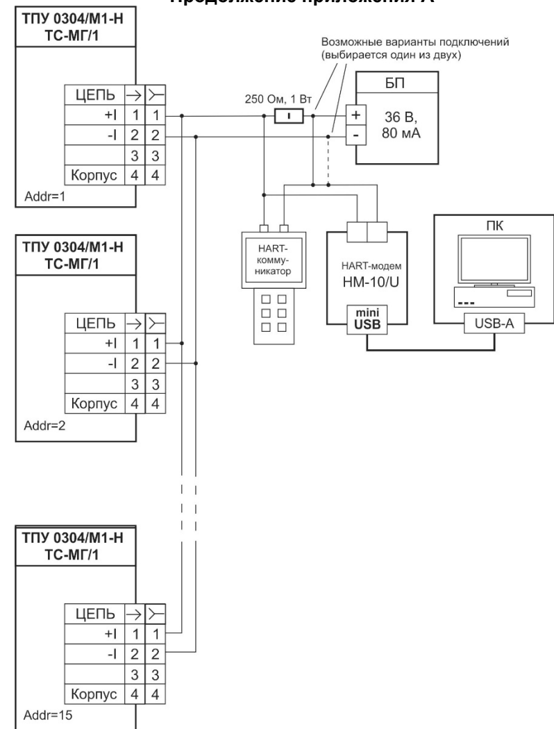
Рисунок А.20 - Схема «многоточечного» (сетевое) подключения ТПУ 0304/M1-H с ТС-МГ/1 с ТС-МГ/1 по HART-протоколу. (Короткий адрес = 1...15)
