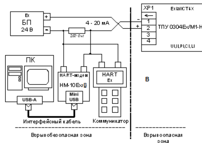
Рисунок А.12 - Схема электрическая подключений ТПУ 0304Ex/M1-H по HART-протоколу через разъем на корпусе термопреобразователя при установке преобразователей во взрывоопасной зоне
