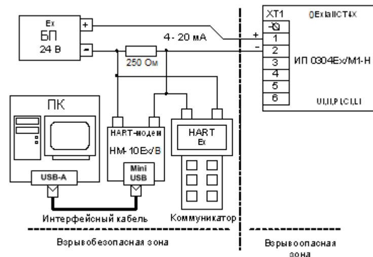
Рисунок А.11 - Схема электрическая подключений ТПУ 0304Ex/M1-H по HART-протоколу через кабельный или сальниковый ввод при установке преобразователей во взрывоопасной зоне
