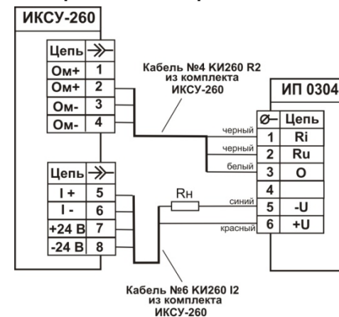
Рисунок А.15 – Схема электрическая подключений ИП 0304/М1-Н и ИКСУ
