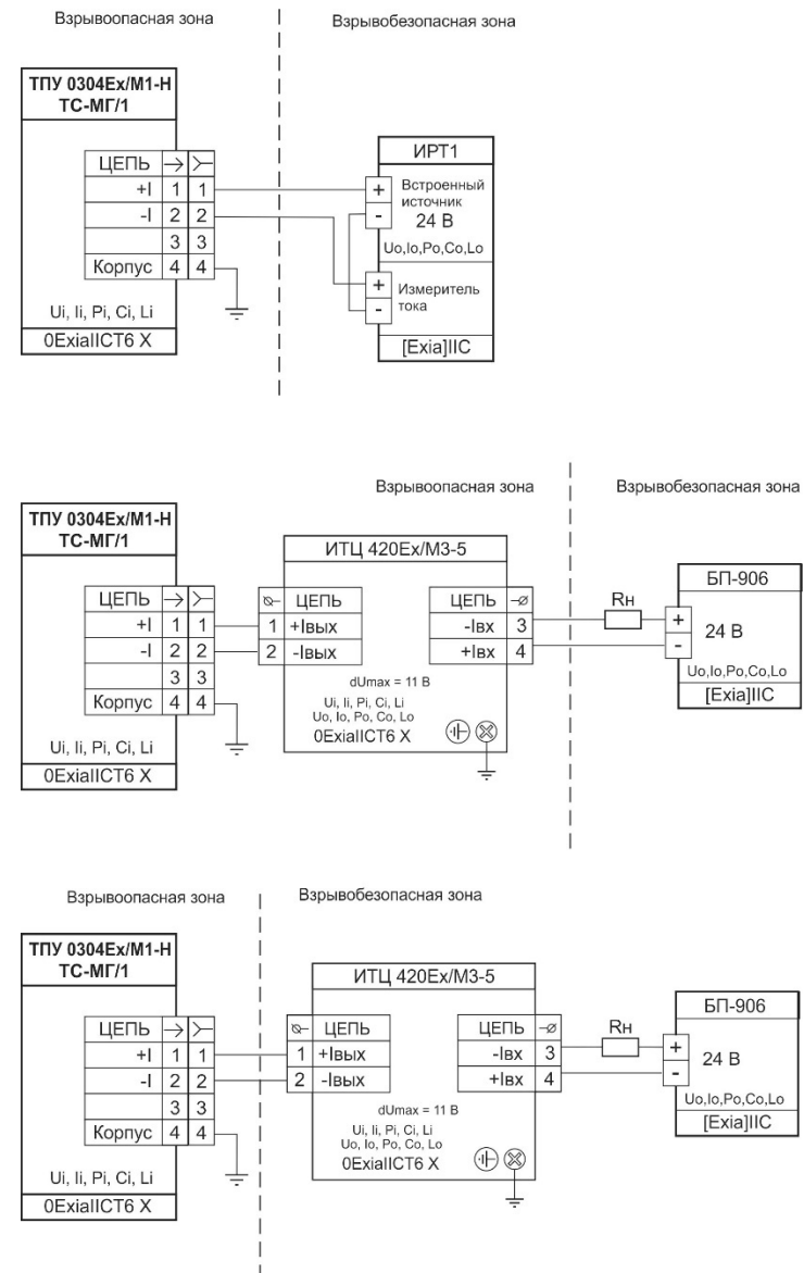
Рисунок А.18 - Схема электрическая подключений ТПУ 0304/M1-H с ТС-МГ/1 по токовой петле 4-20 мА во взрывоопасной зоне
