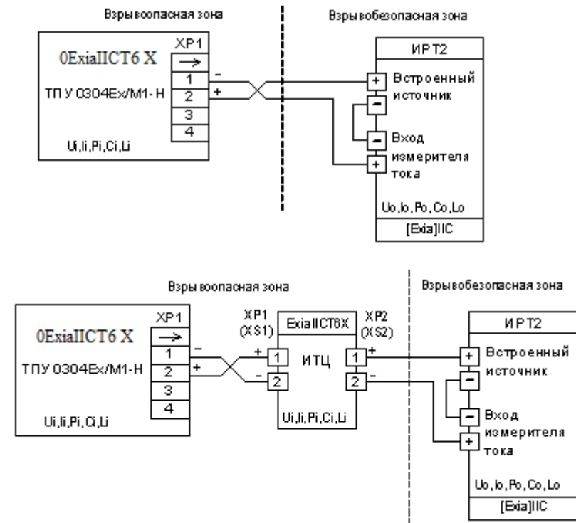
Рисунок А.8 - Схема электрическая подключений ТПУ 0304Ex/M1-N по унифицированному токовому сигналу 4-20 мА через разъём на корпусе термопреобразователя при установке преобразователей во взрывоопасной зоне
