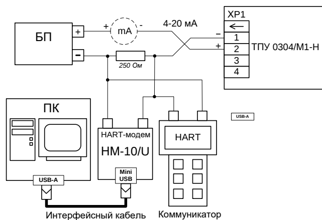
Рисунок А.10 - Схема электрическая подключений ТПУ 0304/М1-Н по HART-протоколу через разъём на корпусе термопреобразователя
