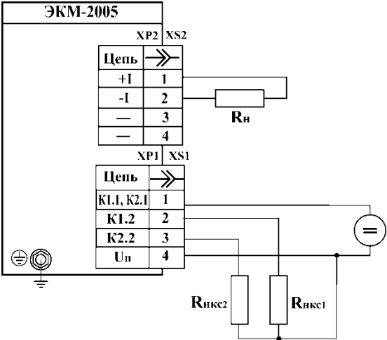
Рисунок 3.4 Схема электрическая подключений ЭКМ-2005 в корпусе АГ-16 без токового выхода с напряжением питания ~ 220 В и = 220 В с гальванически развязанными цепями питания и коммутации
