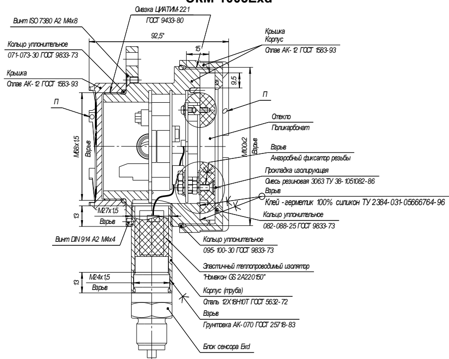
Рисунок А.2 Продолжение приложения А Чертеж обеспечения средств взрывозащиты ЭКМ-1005Exd
