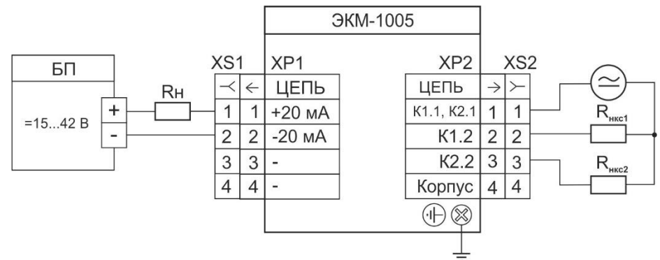
Рисунок 3.3 - Схема электрическая подключений ЭКМ-1005 через кабельный ввод с каналами сигнализации
