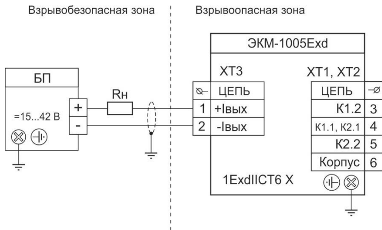
Рисунок 3.5 - Схема электрическая подключений ЭКМ-1005Exd через кабельный ввод без каналов сигнализации
