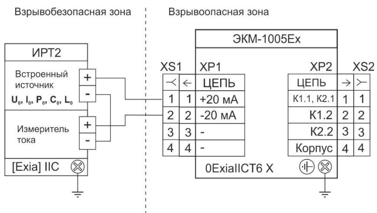
Рисунок 3.8 - Схема электрическая подключений ЭКМ-1005Ex через разъемы GSP 3 M20 (GSP 311) без каналов сигнализации
