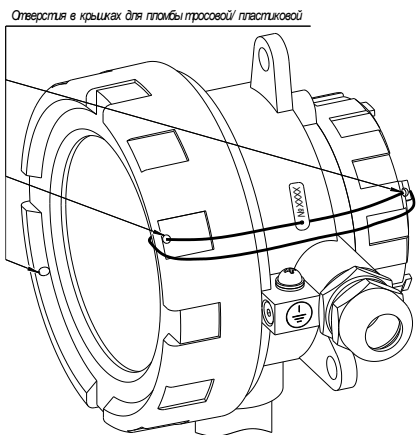
Рисунок А.2 Продолжение приложения А Чертеж обеспечения средств взрывозащиты ЭКМ-1005Exd
