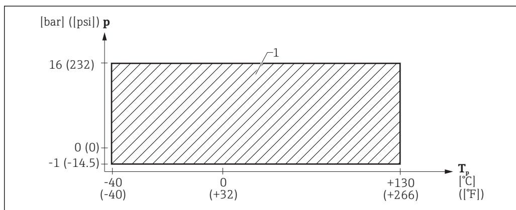
13 FMR60: допустимый диапазон температуры процесса и рабочего давления
