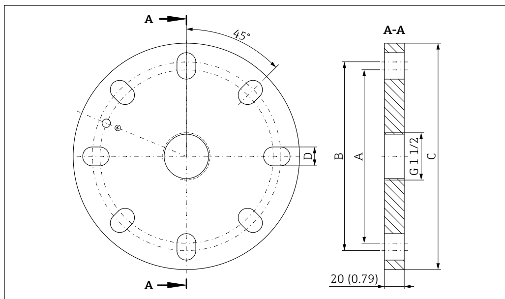
18 Размеры: мм (дюймы)
