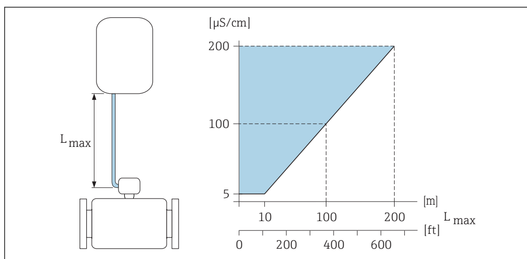
21 Допустимая длина соединительного кабеля
