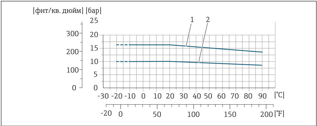
32 Материал присоединения к процессу: нержавеющая сталь (–20 °C (–4 °F)); углеродистая сталь (–10 °C (14 °F))
