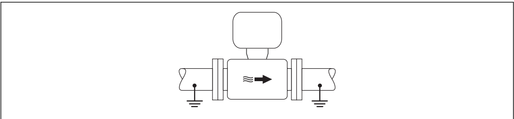
13 Выравнивание потенциалов с использованием измерительной трубки
