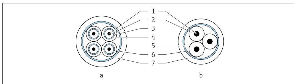
16 Поперечное сечение кабеля
