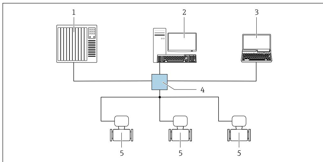
41 Варианты дистанционного управления через сеть EtherNet/IP: топология «звезда»
