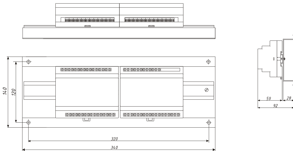
Рисунок 14 – Габаритные размеры блока измерения и блока выходов РВ/8(12)УВ/8(12)Р(Т,С)/(8(12)Р)
