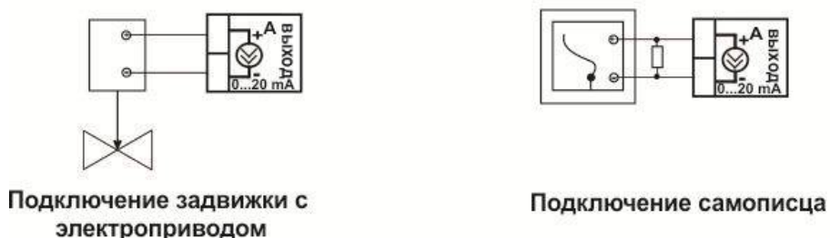
Рисунок 8 – Схемы подключения аналогового выхода
