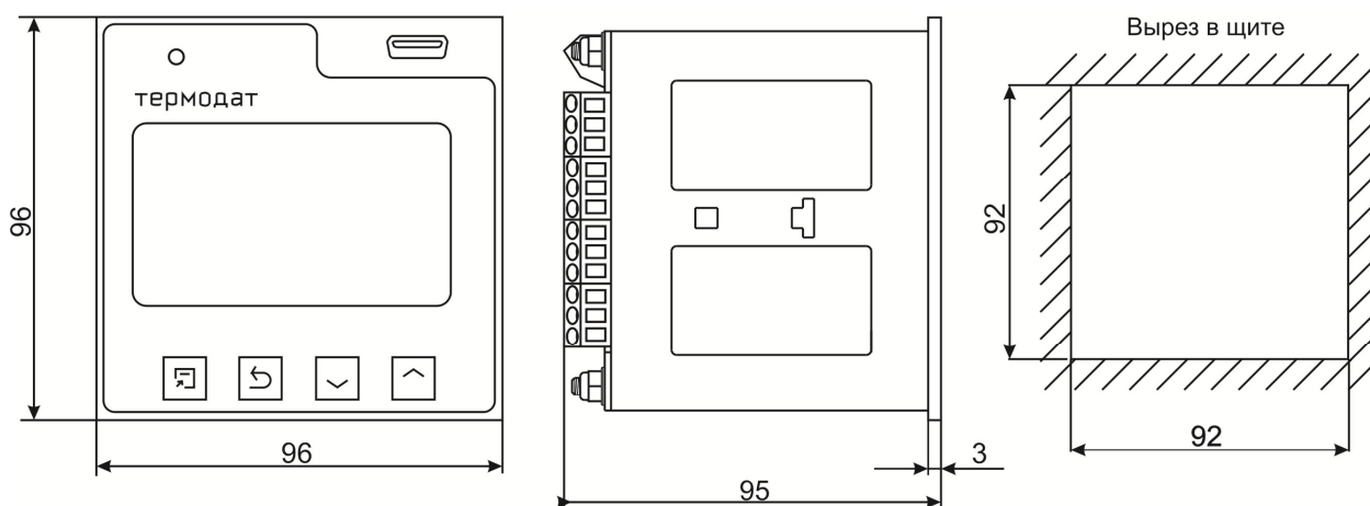
Рисунок 12 – Габаритные размеры основного блока прибора Термодат-25Е6/..../F
