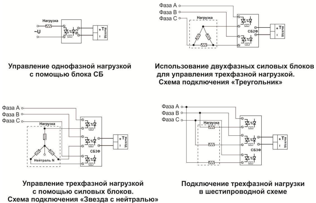
Рисунок 10 – Схемы подключения транзисторного выхода
