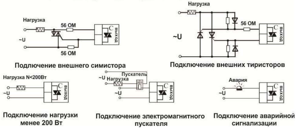
Рисунок 9 – Схемы подключения симисторного выхода
