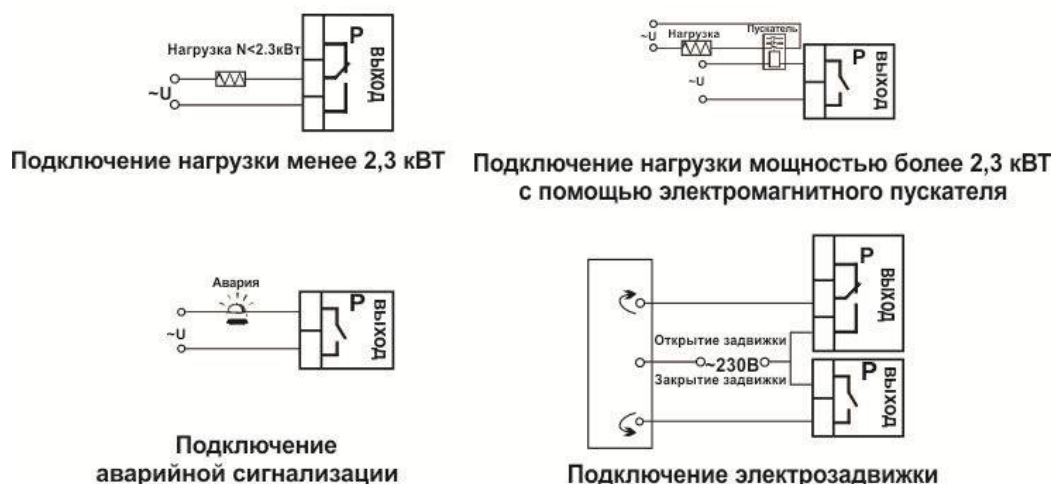
Рисунок 7 – Схемы подключения релейного выхода
