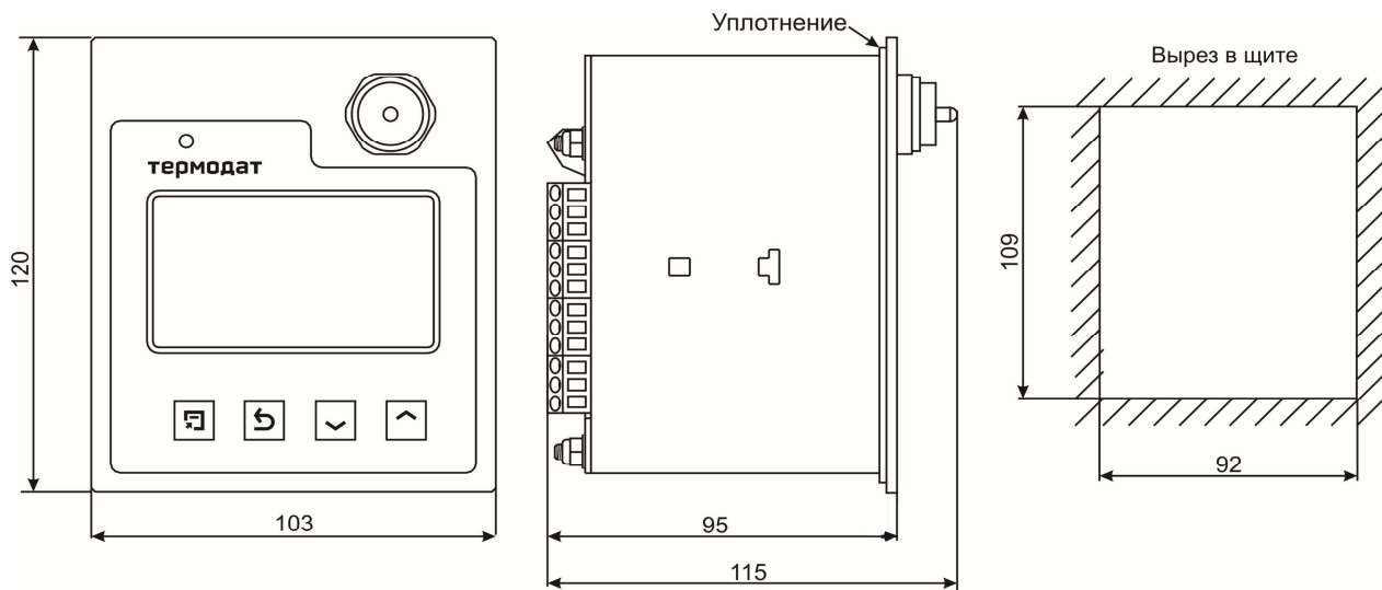
Рисунок 13 – Габаритные размеры основного блока прибора Термодат-25Е6/...../F/IP67
