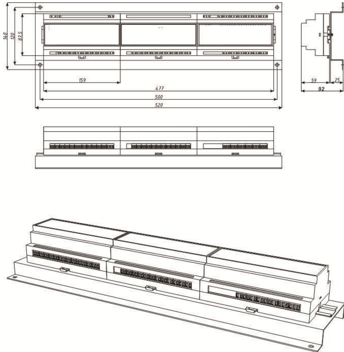
Рисунок 15 – Габаритные размеры блока измерения, блока выходов и блока аналоговых выходов РВ/12УВ/12Р (Т, С)/12Р-12А
