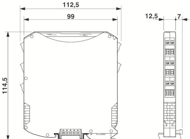
Рисунок 6.1 – Габаритные размеры барьера KA5022Ex-X0 (шинный соединитель не мешает установке барьеров вплотную друг к другу)
