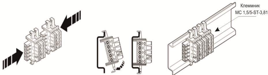
Рисунок 6.3 – Установка шинных соединителей на DIN- рейку
