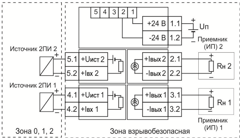
Рисунок 6.3 – Подключение к барьеру источника сигнала с пассивным выходом с двухпроводной схемой подключения
