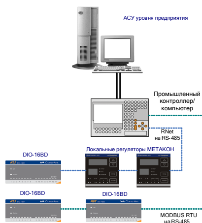
Рисунок 1.1 – MDS-модули в структуре распределенной АСУТП
