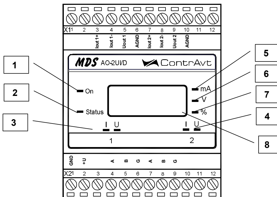
Рисунок 4.1 – Внешний вид модуля со стороны передней панели
