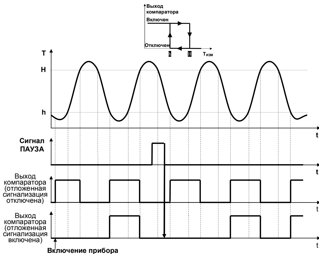
Рисунок 5.17 – Графики, показывающие работу компаратора при отключенной и включенной отложенной сигнализации
