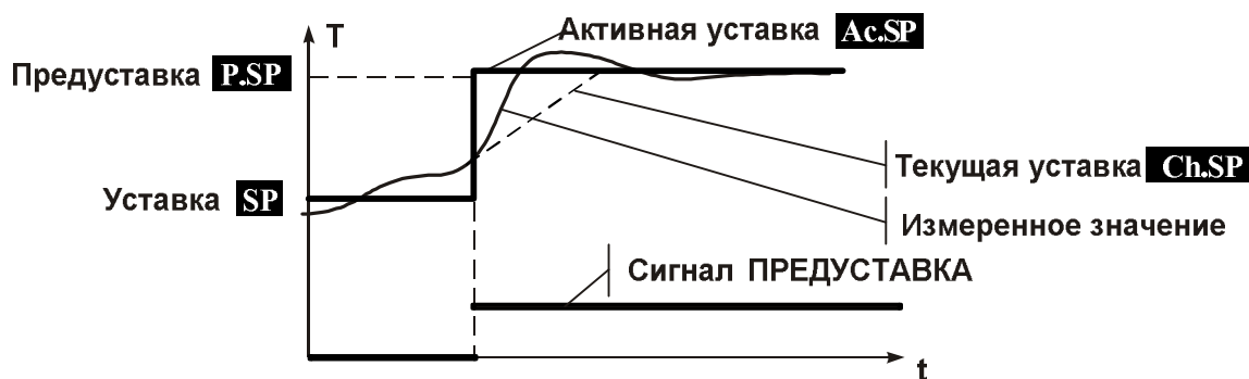
Рисунок 5.3 – Уставки регулятора
