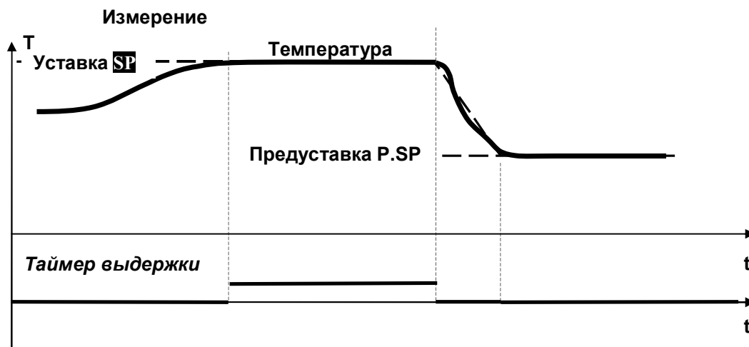
Рисунок 5.15 – Вариант 3 работы регулятора по окончании времени выдержки
