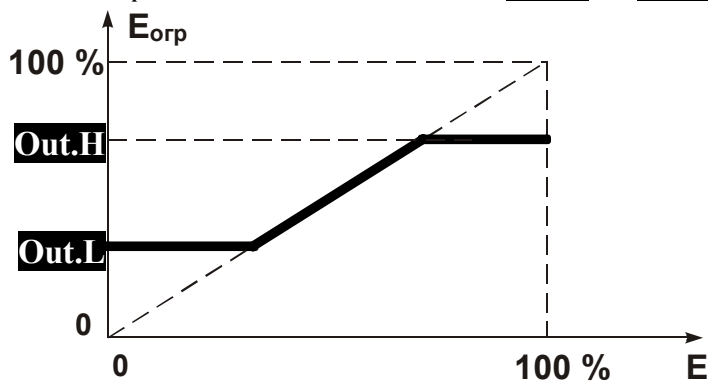
Рисунок 5.5 – Ограничение сигнала управления
