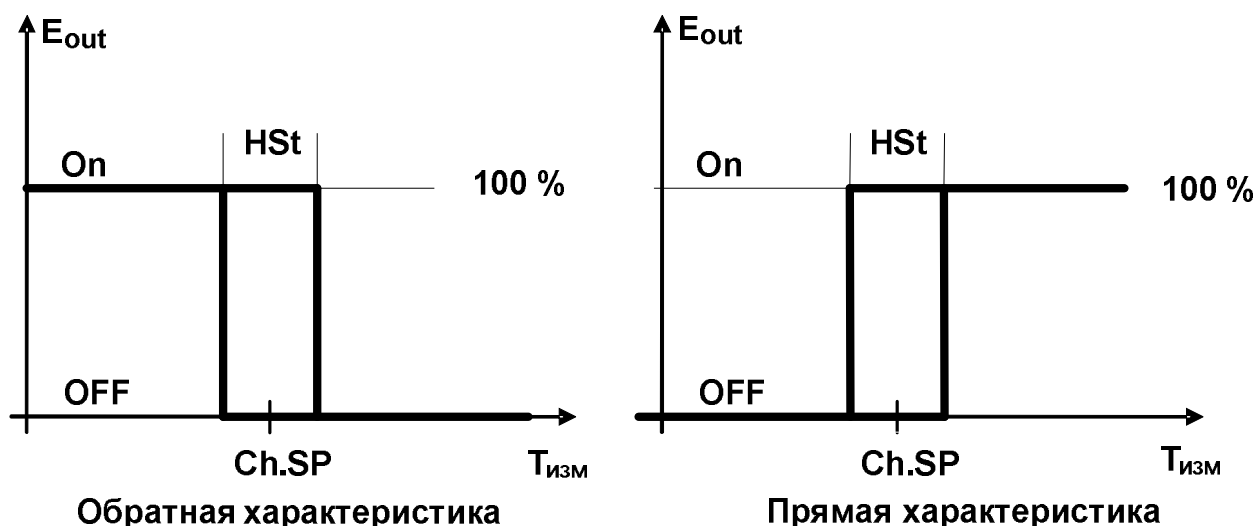
Рисунок 5.8 – Работа позиционного регулятора
