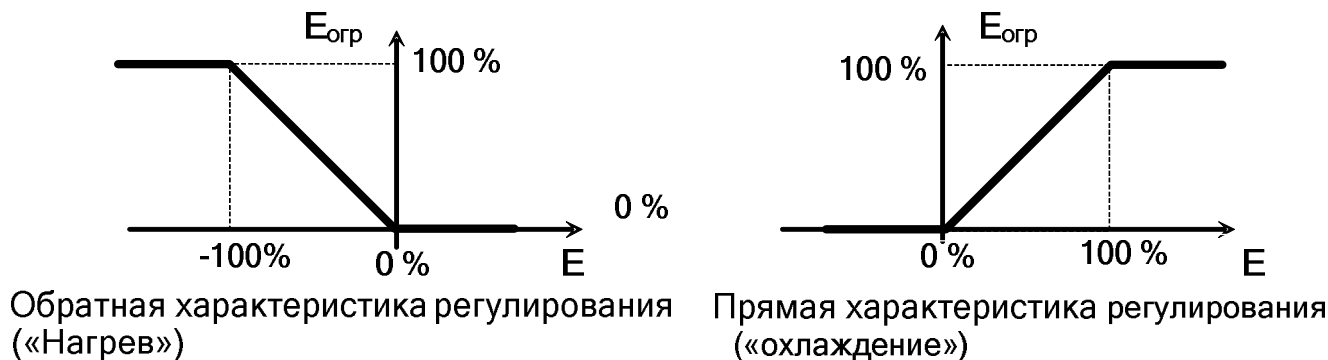
Рисунок 5.4 – Зависимость сигнала управления от рассогласования.
