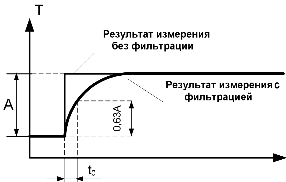
Рисунок 5.9 – График, показывающий влияние цифровой фильтрации результата измерения
