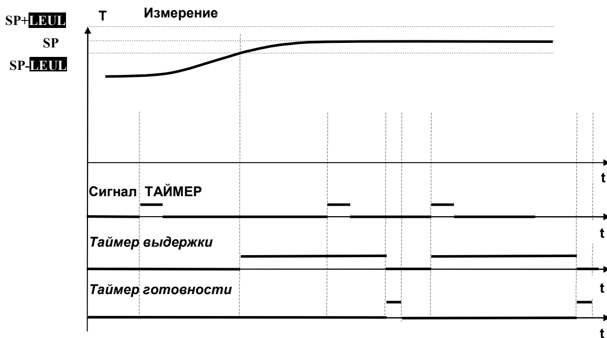
Рисунок 5.12 – Диаграмма работы таймера выдержки с условным запуском сигналом ТИЙМЕР по уровню измеренного параметра
