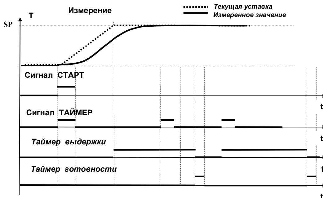
Рисунок 5.13 – Диаграмма работы таймера выдержки с условным запуском сигналом ТАЙМЕР по уровню текущей уставки
