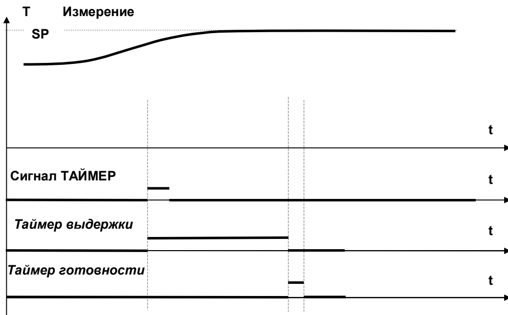
Рисунок 5.11 – Диаграмма работы таймера выдержки с безусловным запуском сигналом ТИЙМЕР
