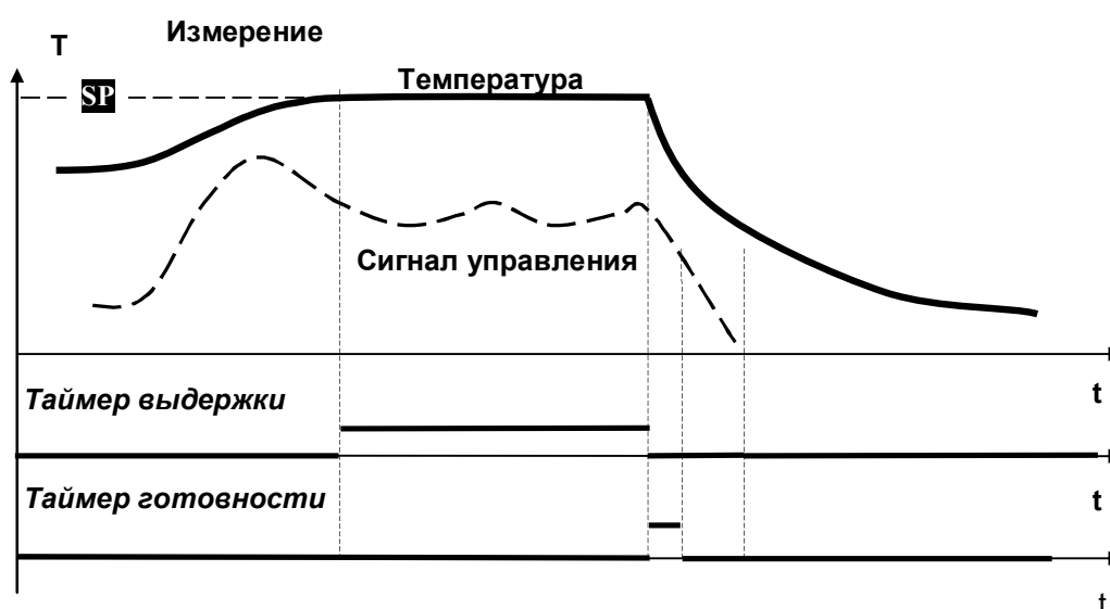
Рисунок 5.14 – Вариант 2 работы регулятора по окончании времени выдержки
