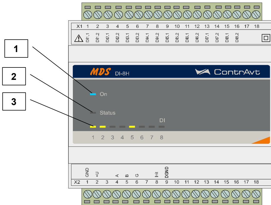
Рисунок 4.1 – Вид модуля со стороны передней панели
