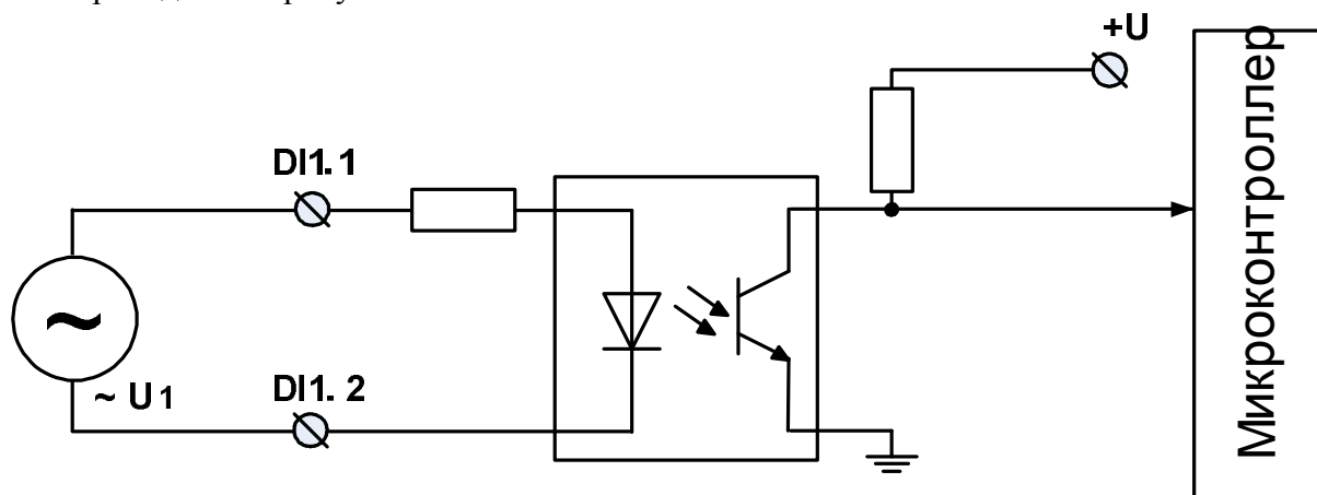
Рисунок 5.2 – Подключение к модулю сигналов напряжения переменного тока
