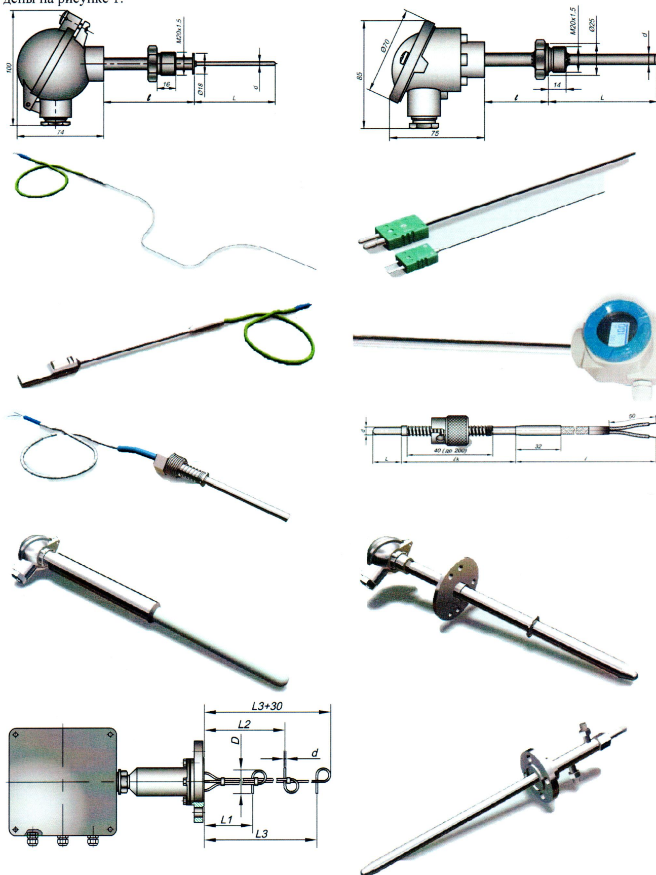
Рисунок 1 – Датчики температуры КТХА, КТНН, КТХК, КТЖК, КТМК
