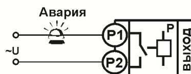
Подключение аварийной сигнализации
