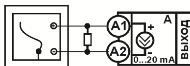
Подключение самописца
