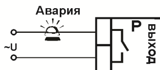
Подключение аварийной сигнализации
