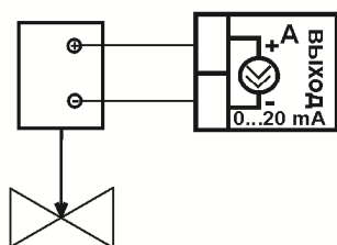
Подключение задвижки с электроприводом
