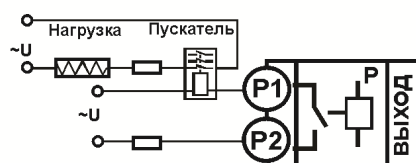
Подключение нагрузки мощностью более 1,5 кВт с помощью электромагнитного пускателя
