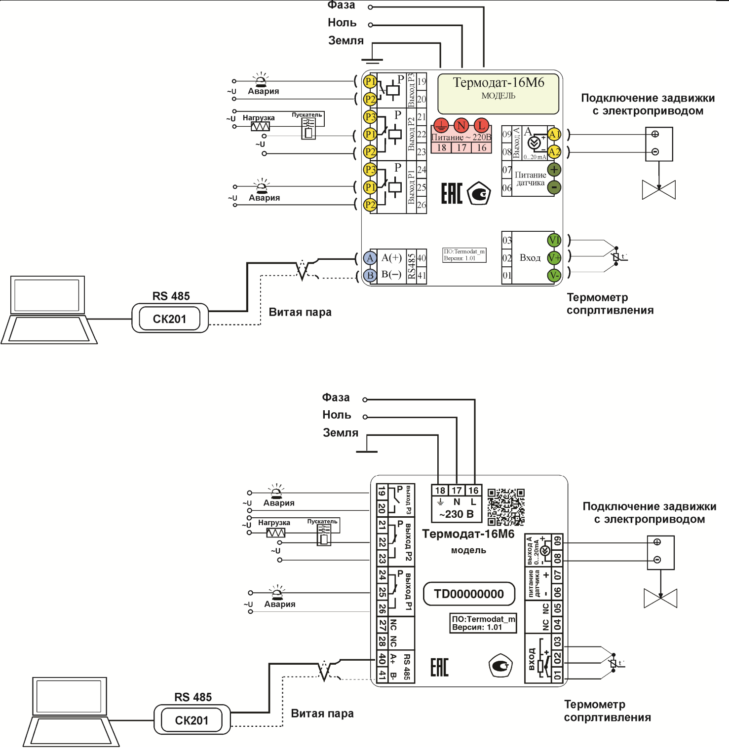
Типовая схема подключения прибора
