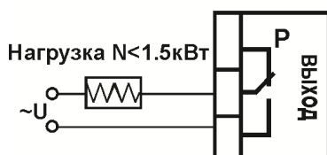
Подключение нагрузки менее 1,5 кВт
