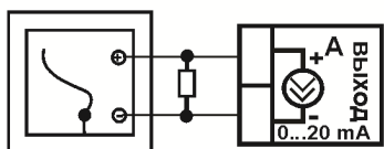
Подключение самописца
