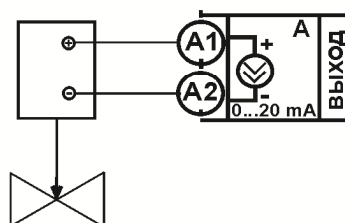
Подключение задвижки с электроприводом
