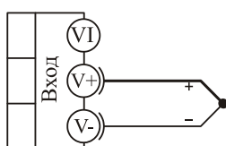
термопара
