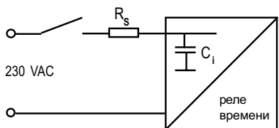
Ограничение тока при ёмкостной нагрузке при подключении электронного реле времени (рис. 4)
