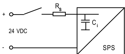
Ограничение тока при ёмкостной нагрузке (рис. 3)
