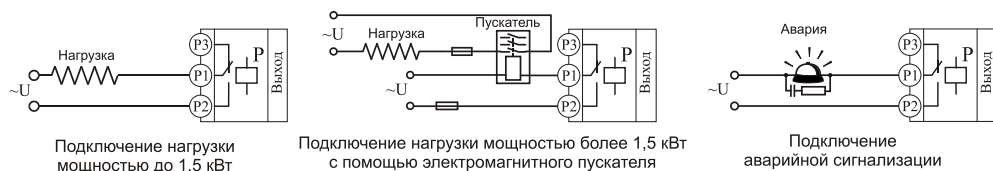
Рис.1 Использование релейного выхода
