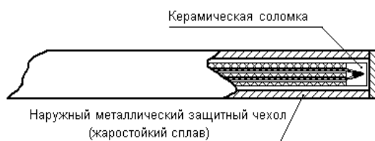
Конструкция рабочей зоны термопреобразователей ТППТ(ТПРТ) 01.06, D = 7
