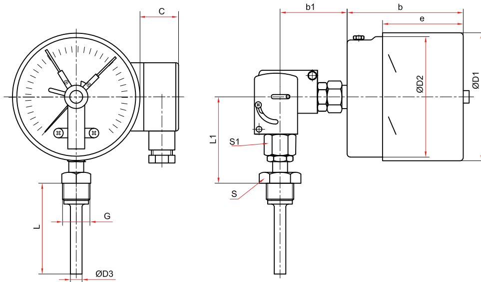
Универсальное присоединение (Ø100 мм)
