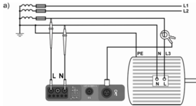
Вариант подключения токовых клещей
