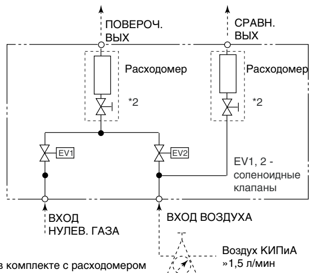
Блок автокалибровки ZR40H
