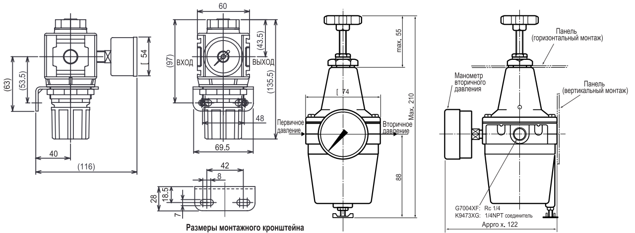
Размеры монтажного кронштейна
