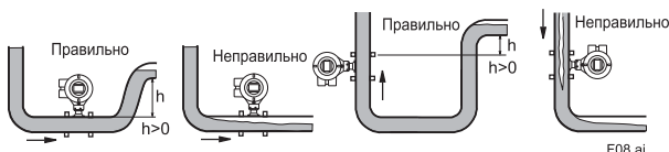
Конфигурация трубопровода
