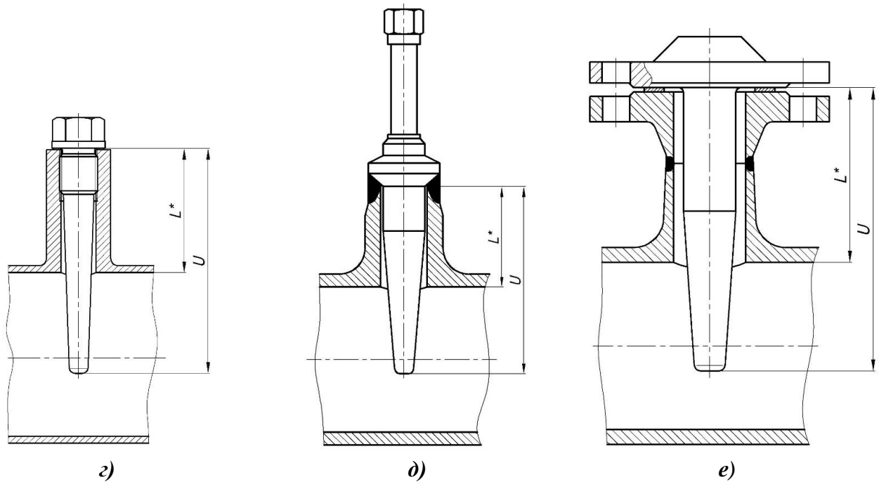
Рис. 7 — Примеры установки гильз защитных на трубопровод
